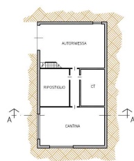
PIANTA PIANO INTERRATO
